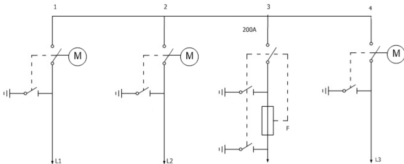
Fig. 1 Schema monofilară
