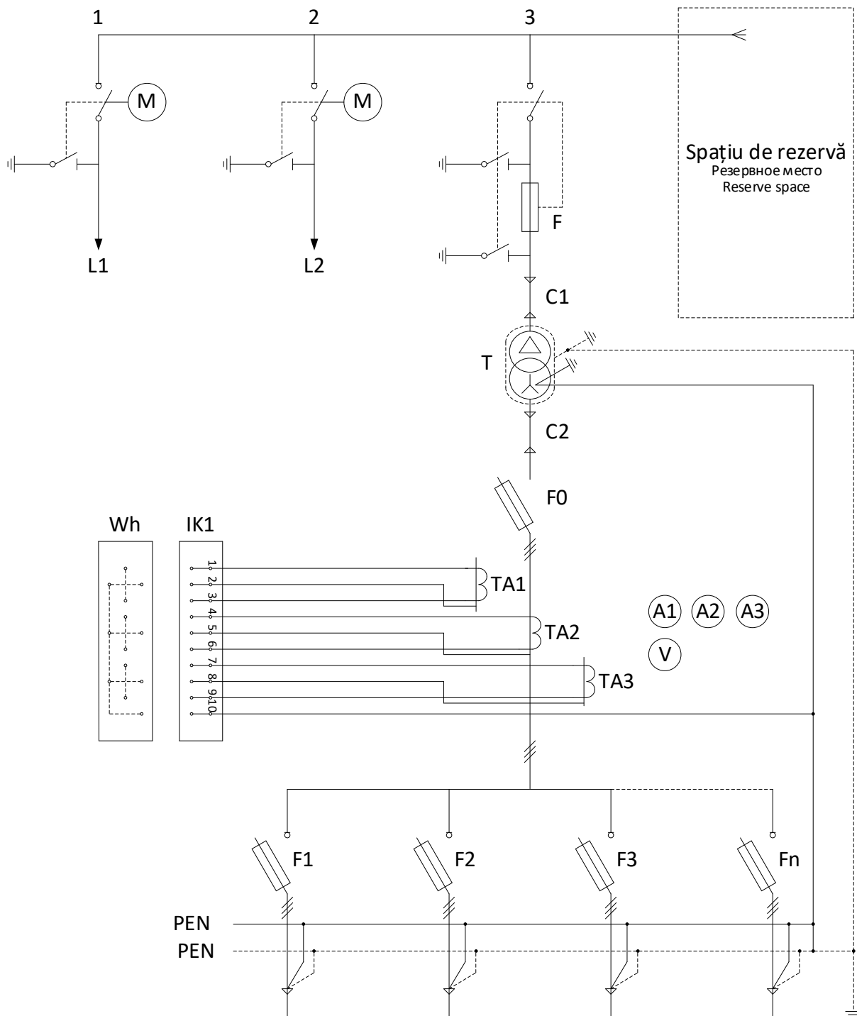
Fig. 1 Schema monofilară
