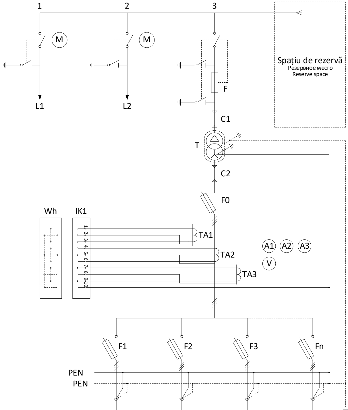
Fig. 1 Schema monofilară
