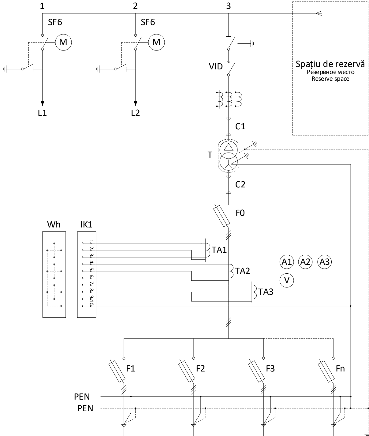
Fig. 1 Schema monofilară
